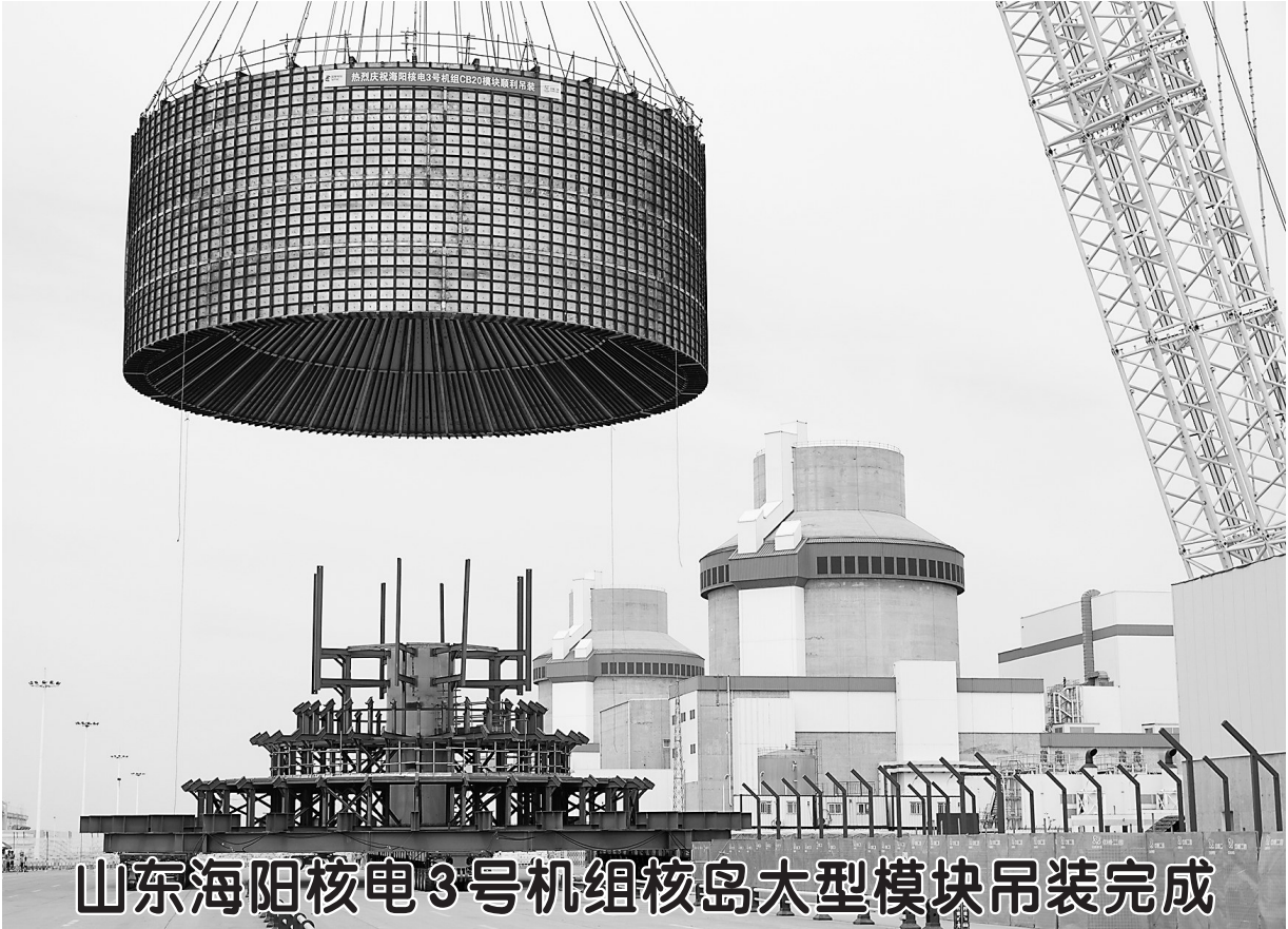
这是8月4日拍摄的山东海阳核电3号机组核岛CB20模块吊装现场。当日,国家电投山东海阳核电站3号机组核岛CB20模块顺利吊装就位,标志着该机组大型模块全部吊装完成,开始进入设备安装调试阶段。据了解,建设中的海阳核电3、4号机组是国家“十四五”规划重点项目,计划2027年全面投运。
