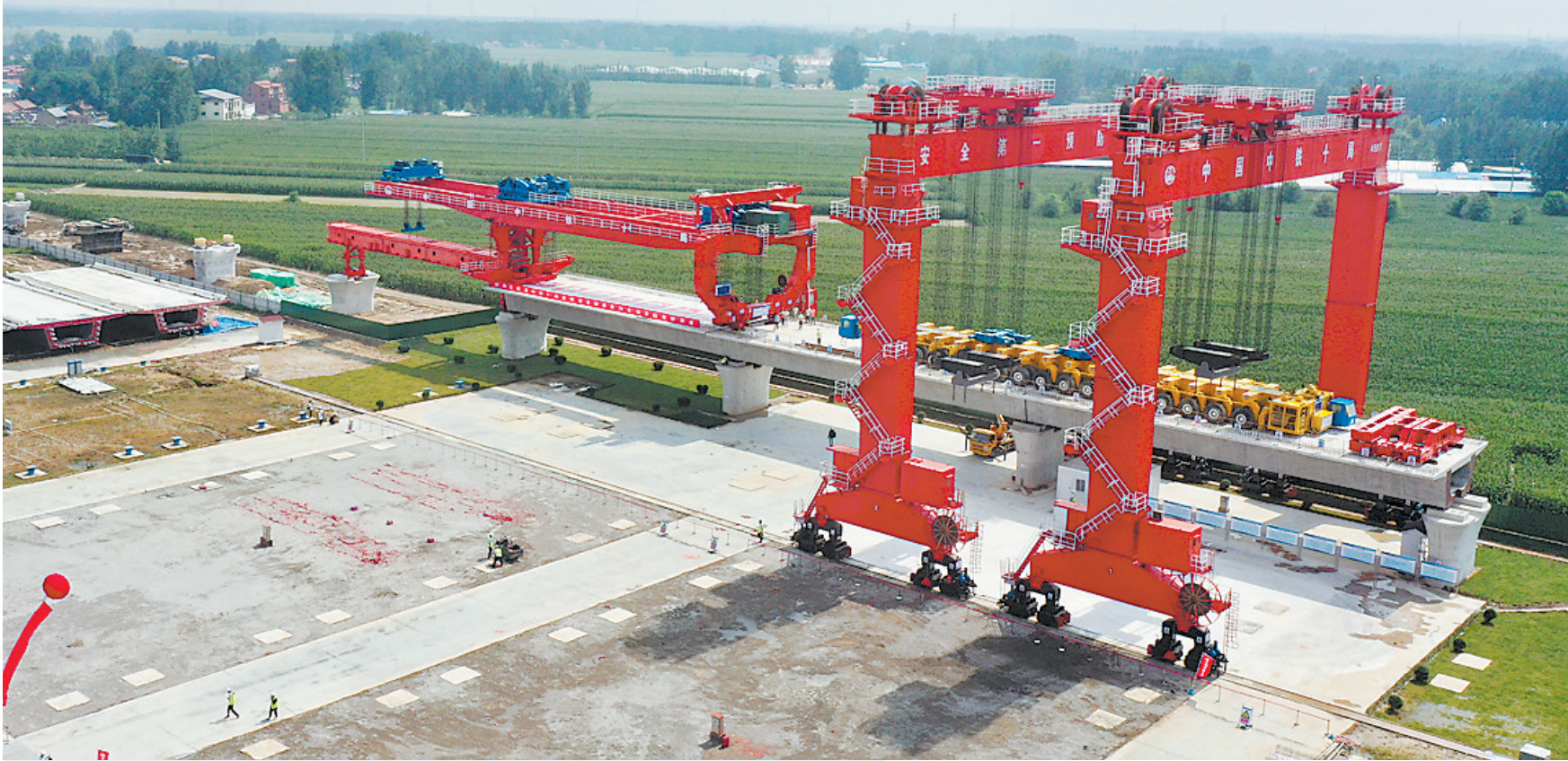
▲▼雄商高铁菏泽段箱梁架设现场。
